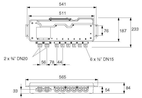
Mått på blandarlådan i mm.
