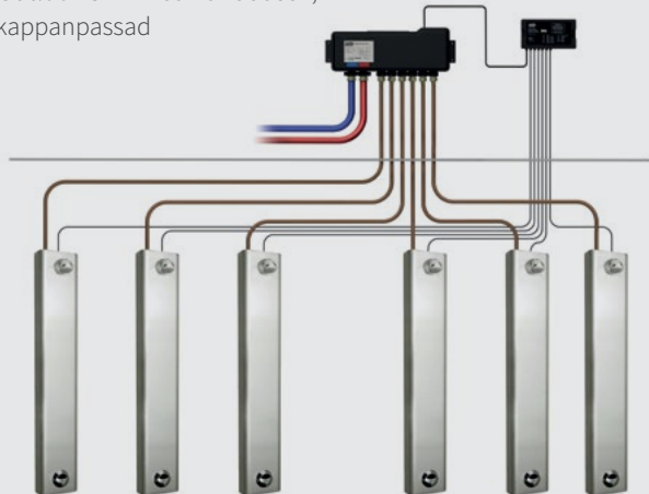
DP3 Outlook anslutna till Rada Outlook-systemet.
